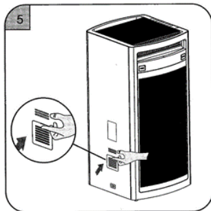
5- Placer le nouveau module dans son logement et refermer le couvercle.
