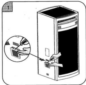
1- Faire levier sur le couvercle du capteur avec un tournevis plat adapté à la taille de la fente.
